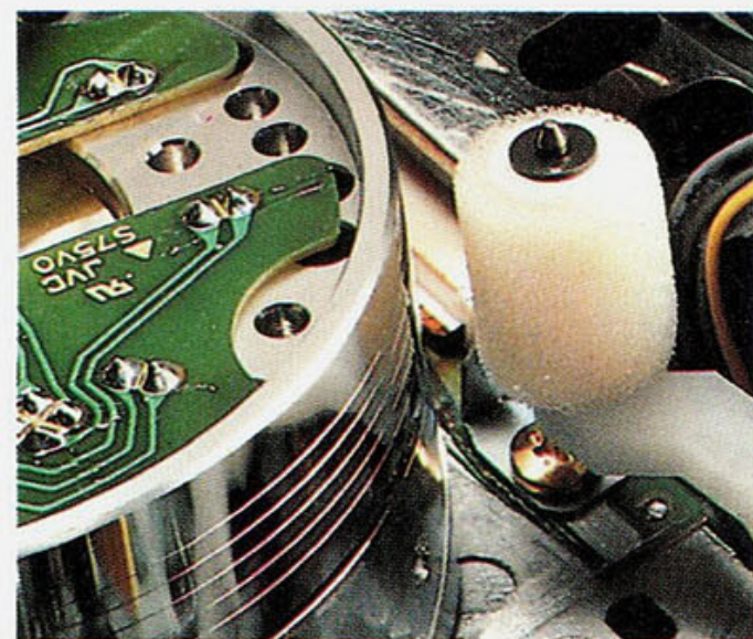
Cada vez que a fita é colocada ou retirada dos novos vídeos JVC, o sistema de Auto-Limpeza das cabeças é acionado.
