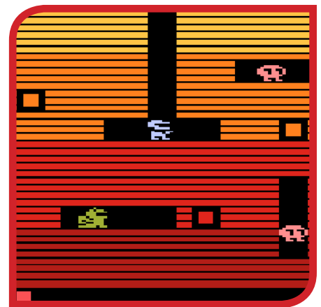
DIG DUG
