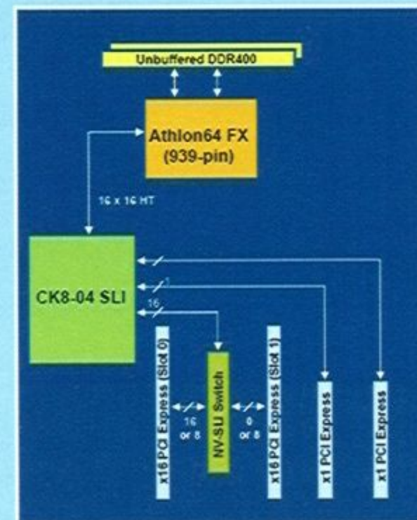
nVidia SLI 架構圖
