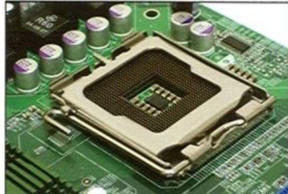
661FM3-L 的 CPU 插座採用 Socket T 規格，支援 LGA775 處理器。
