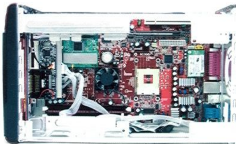
這是取下電源供應器與磁碟機框架後，所見到的 MEGA 865 內裝情形。
