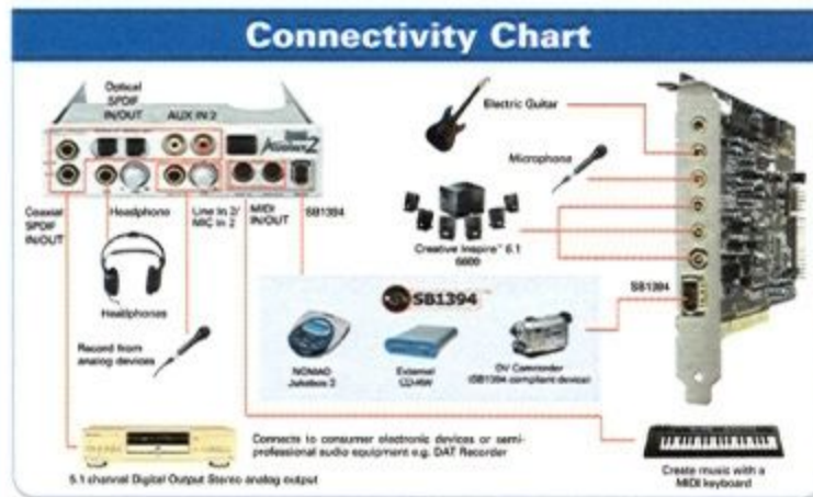
前置面板 Audigy2 Drive 連接設備示意圖
