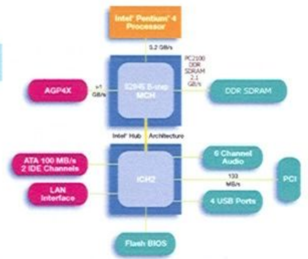
1845D 晶片組工作模式架構圖
