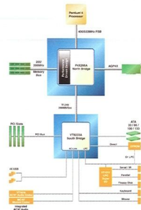
VIA P4X266A 晶片組工作模式架構圖
