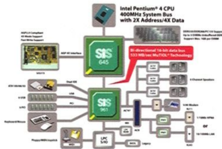
SiS645 晶片組工作模式架構圖
