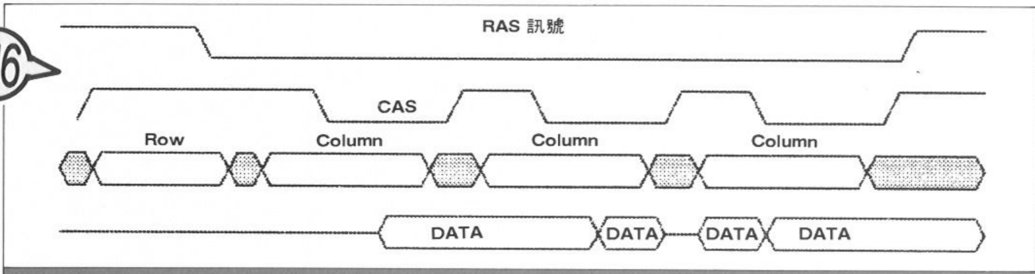
EDO RAM 的時序圖，本圖僅為表達 EDO RAM 的資料時間所佔比例比一般 DRAM 長，其它訊號並未列入
