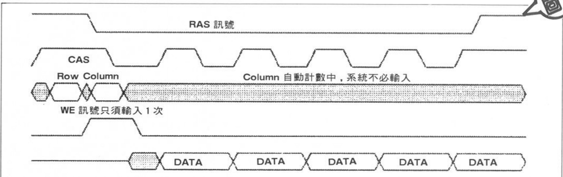
EDO RAM 爆發模式下的時序圖，此時行位址 (Column) 只輸入一次，之後資料會以 20 奈秒為一個週期不斷向外送
