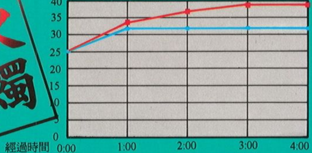
硬碟抽取盒溫昇測試 (SCSI)
