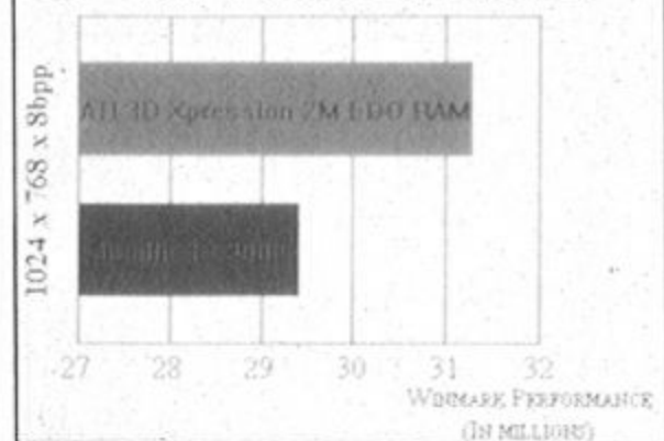
2D 顯示速度比較圖
