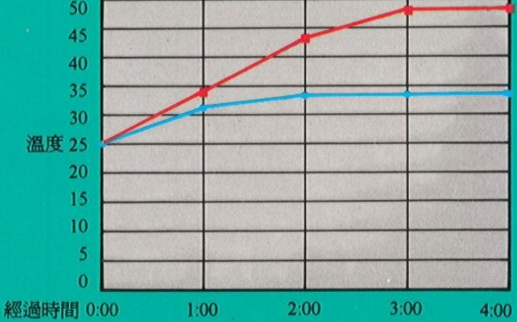
硬碟抽取盒溫昇測試 (SCSI)
