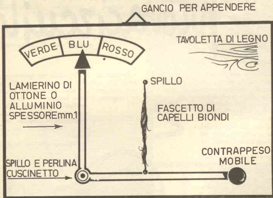
IGROMETRO A CAPELLO
