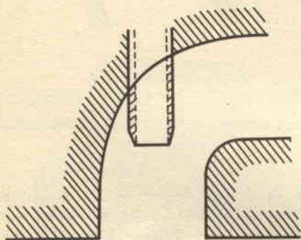
Fig. 1: Condotto con la strozzatura dovuta alla guida della valvola.
