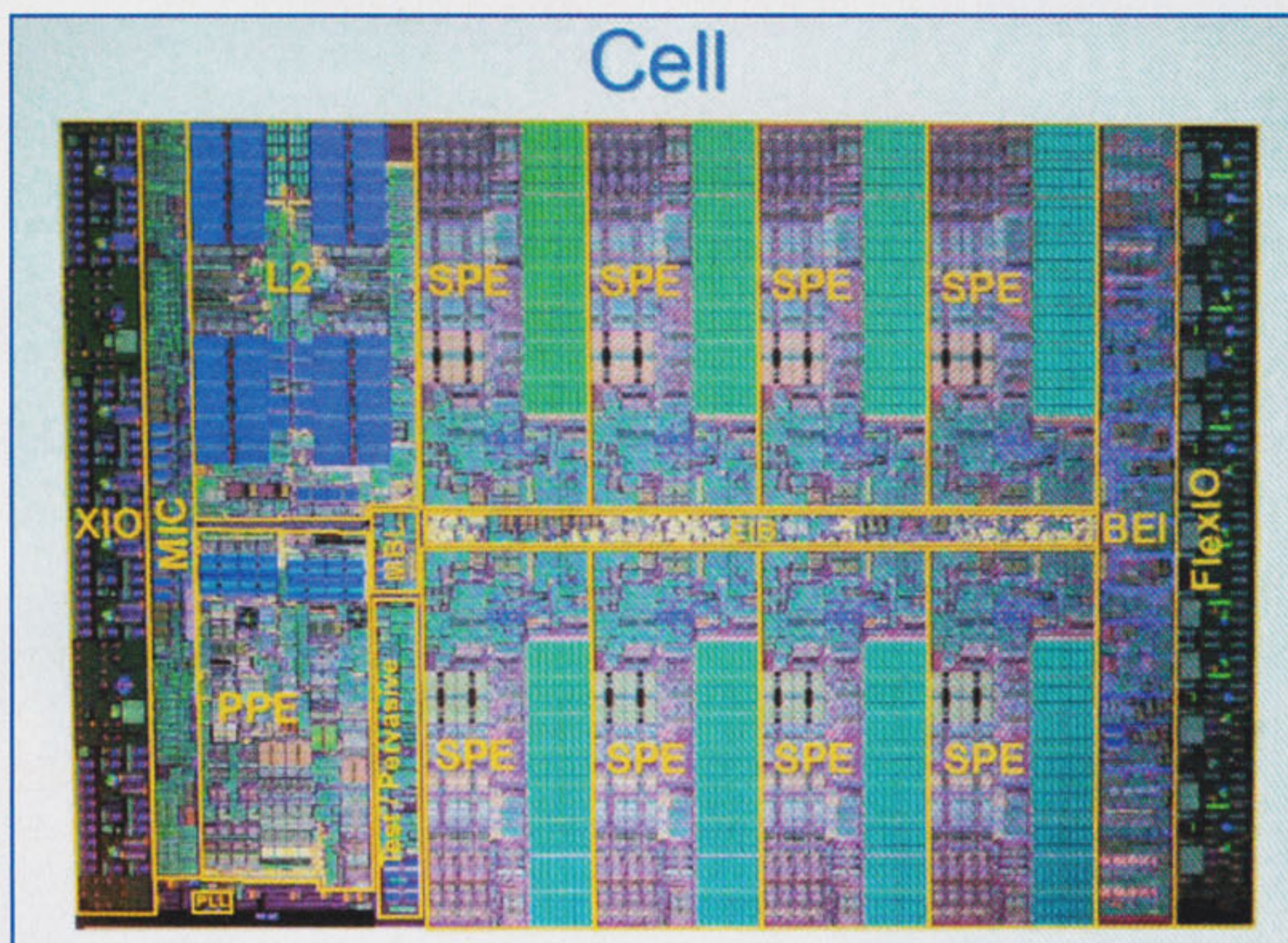
Slide mostra cada um dos componentes e os nove núcleos (PPE e SPE) do chip.
