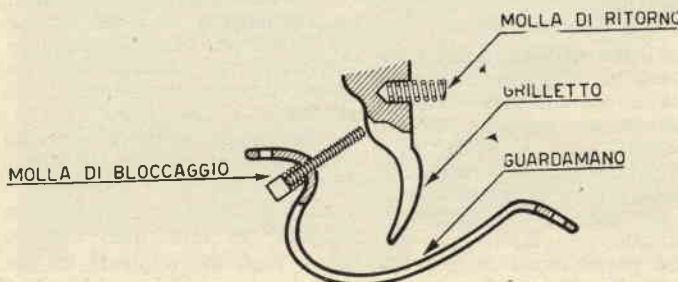
Fig. 5. — Applicazione delle viti di regolazione scatto
