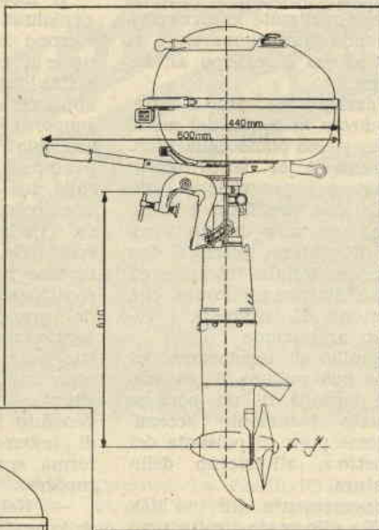
Fig. 3 - Il MOSCONE viene fornito a richiesta con o senza prolunga.
