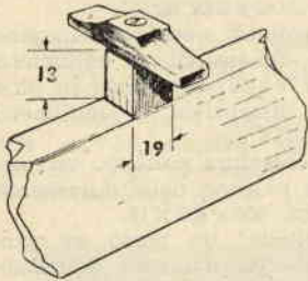
Fig. 22. - Tavolato e particolare levetta fissaggio assicelle mobili.
