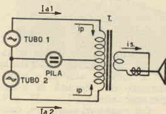
Fig. 7. — Circuito equivalente di uno stadio push-pull.
