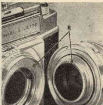
Fig. 12. - Dal dettaglio d'attacco dell'obiettivo ci si potrà render conto come l'operazione richieda una certa quale attenzione, al fine di non rovinare nè attacco, nè lamelle dell'otturatore.
