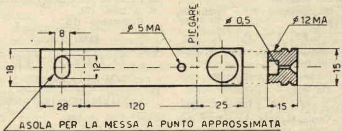
Fig. 2. — Supporto oculare.
