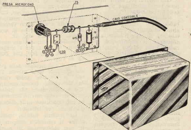
Fig. 3 - La presa del microfono, C30, J5, R15 e C15 dovranno risultare schermati e allo scopo verranno protetti da una custodia metallica.
