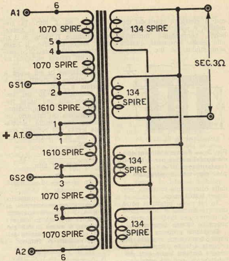
Fig. 8. — Trasformatore Hi-Fi.
