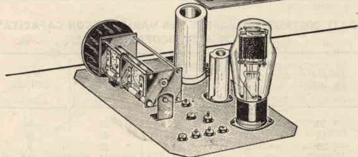
Fig. 7 - La parte superiore del VFO risulta racchiusa da una scatola in lamierino forato, o in lamiera stirata.
