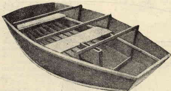
Fig. 14. - Scafo rimosso dalla sagoma di montaggio, con traverse di irrigidimento rimesse in posizione.
