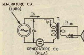
Fig. 4. — Circuito equivalente di uno stadio di potenza. I_a = corrente continua anodica i_p = corrente alternata primaria prodotta dai suoni i_s = corrente alternata secondaria, che fa vibrare il cono dell'altoparlante percorrendo la bobina mobile.
