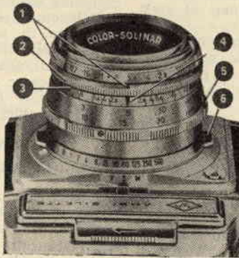
Fig. 16. - Montaggio obiettivo.
