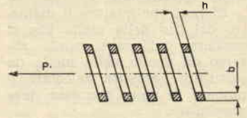
Fig. 9. — Molla a sezione rettangolare.
