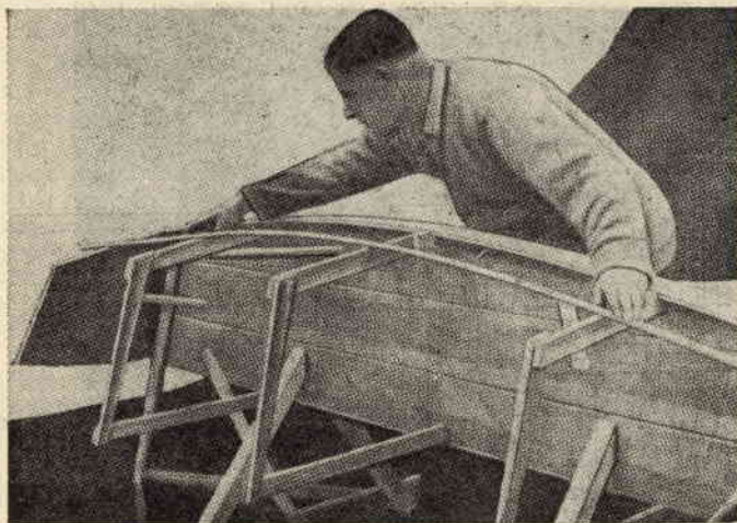
Fig. 11. - Metodo di controllo allineamento ordinate e pannelli.
