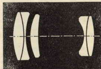
Fig. 15. - Obiettivo tele.
