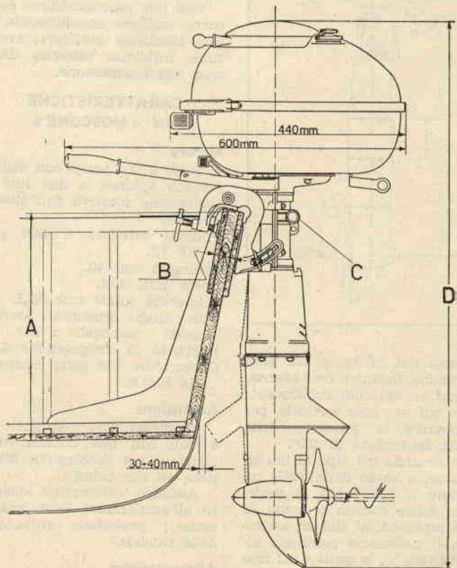
Fig. 2. — Ancoramento del MOSCONE allo specchio di poppa dello scafo.
