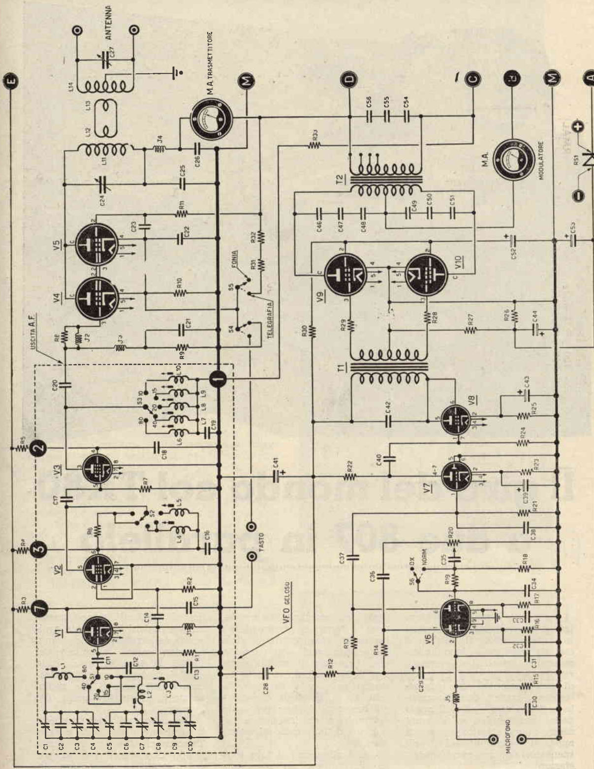
Fig. 1 - Schema elettrico del trasmettitore, fatta eccezione dell'alimentatore.
