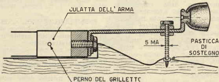
Fig. 3. — Disposizione dell'oculare.
