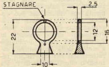
Fig. 1. — Reticolo.
