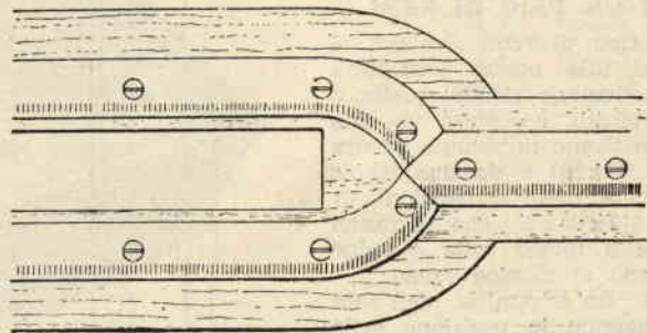
Fig. 18. - Irrobustimento asse di chiglia e feritoia coltello.
