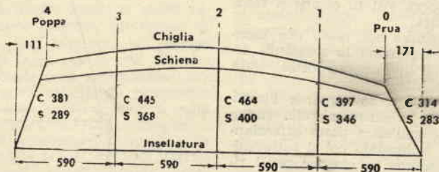
Fig. 2. - Sezione longitudinale del battello.
