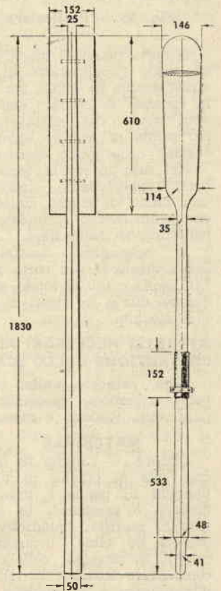
Fig. 24. - Forme e dimensioni remi.
