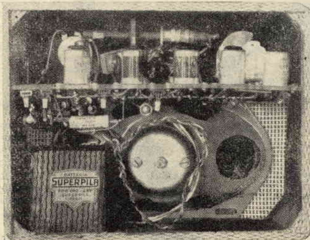
Fig. 3. - Allogamento del complesso all'interno della custodia (vista posteriore).
