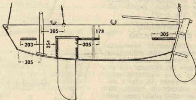
Fig. 4. - Spaccato longitudinale del battello.
