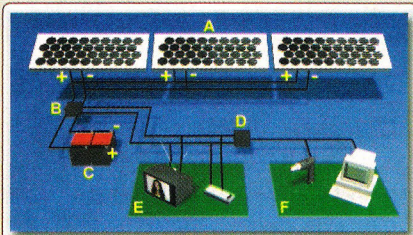
Figura 2 - Sistema da Heliodinâmica ( www.heliodinamica.com.br ) para uso de energia solar com suas placas solares.
