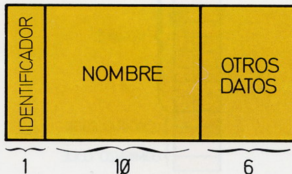
Los diecisiete bytes de un header, se distribuyen en: identificador, nombre y datos diversos.
