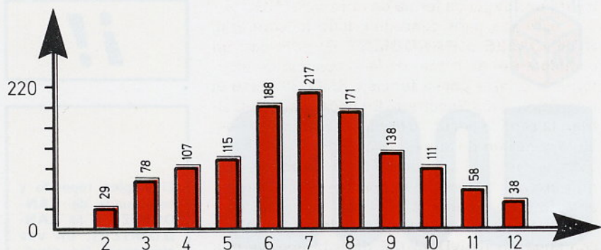
La gráfica correspondiente a las ocurrencias en el lanzamiento de dos dados, adopta la forma conocida como «campana de Gauss».
