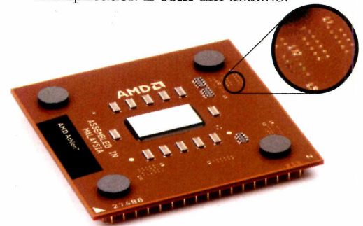
Chip Athlon: Destaque para os fusíveis que devem ser unidos com grafite
