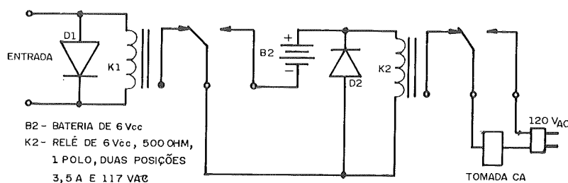
Figura 2A — Circuito de interface e controle para eletrodomésticos e lâmpadas.
