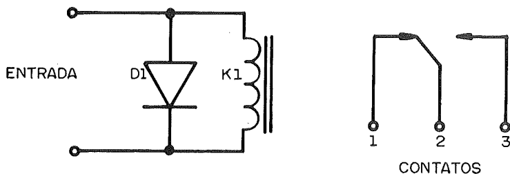
Figura 1 — Circuito de interface utilizando um relé
