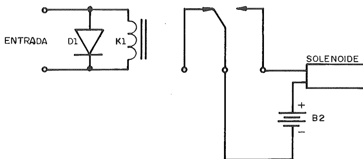
Figura 2B — Circuito de interface e controle para solenóides
