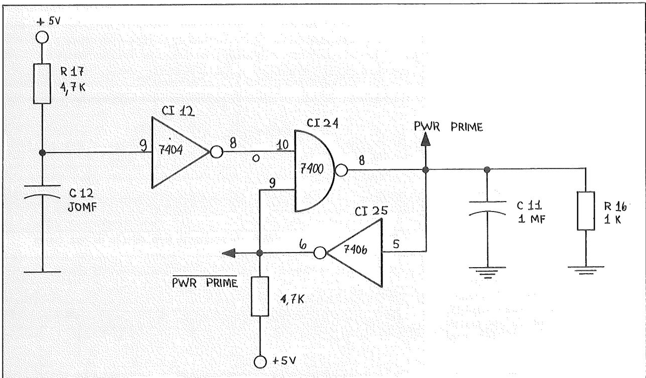
FIGURA 5 — Circuito gerador do sinal PWR PRIME
