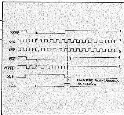
FIGURA 3 — Diagrama de tempo da condição de preparação
