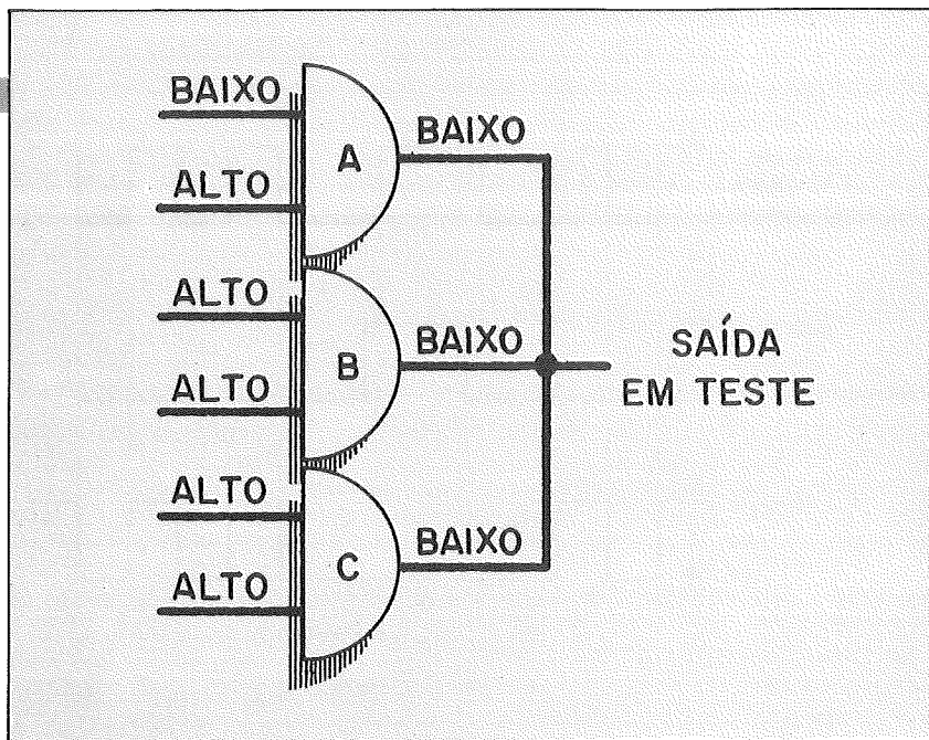
FIGURA 3 — Ligação Wire-And
