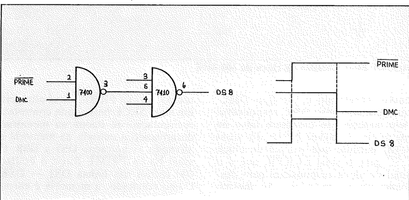
FIGURA 4C- Geração do caractere falso DS8
