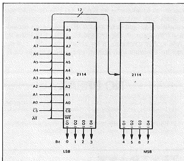
Figura 2B — Organização 1K x 8 Utilizando Duas 2114
