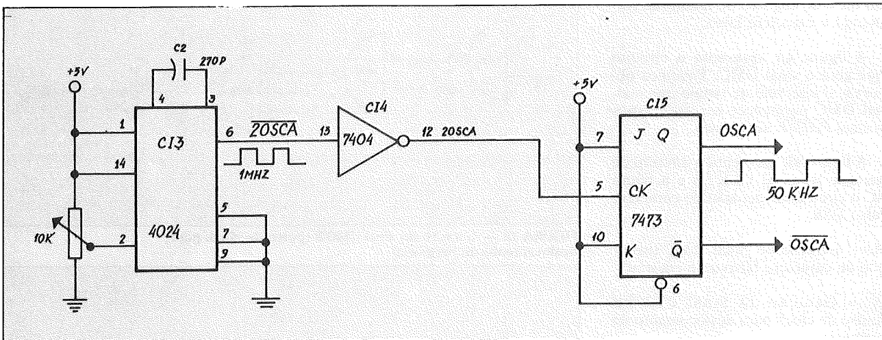
FIGURA 2B — Gerador de clock de 500 KHZ
