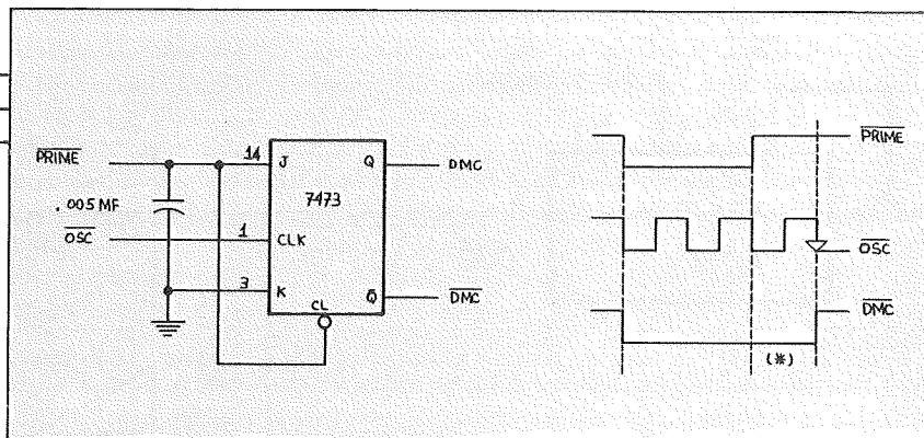
Figura 4A — Geração do sinal DMC (inserção de caractere falso na memória)
