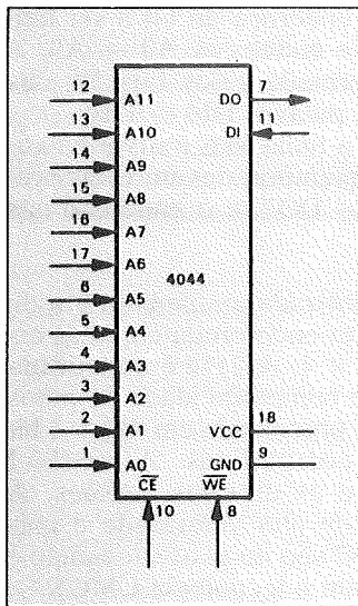
Figura 3A — Configuração dos Pinos
