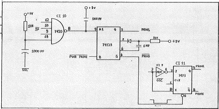
FIGURA 6 — Geração da condição de preparação pela seleção da impressora
