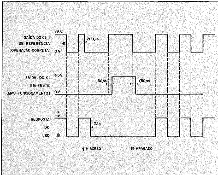
FIGURA 2 — Comparação das respostas dos CIs
