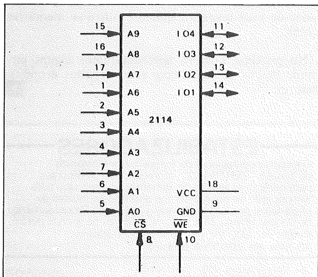
Figura 2A — Configuração dos Pinos
