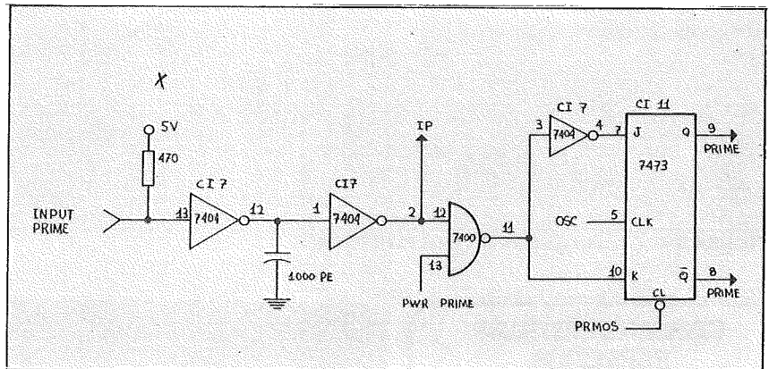
FIGURA 7 — Geração da condição de preparação pelo sinal INPUT PRIME externa
