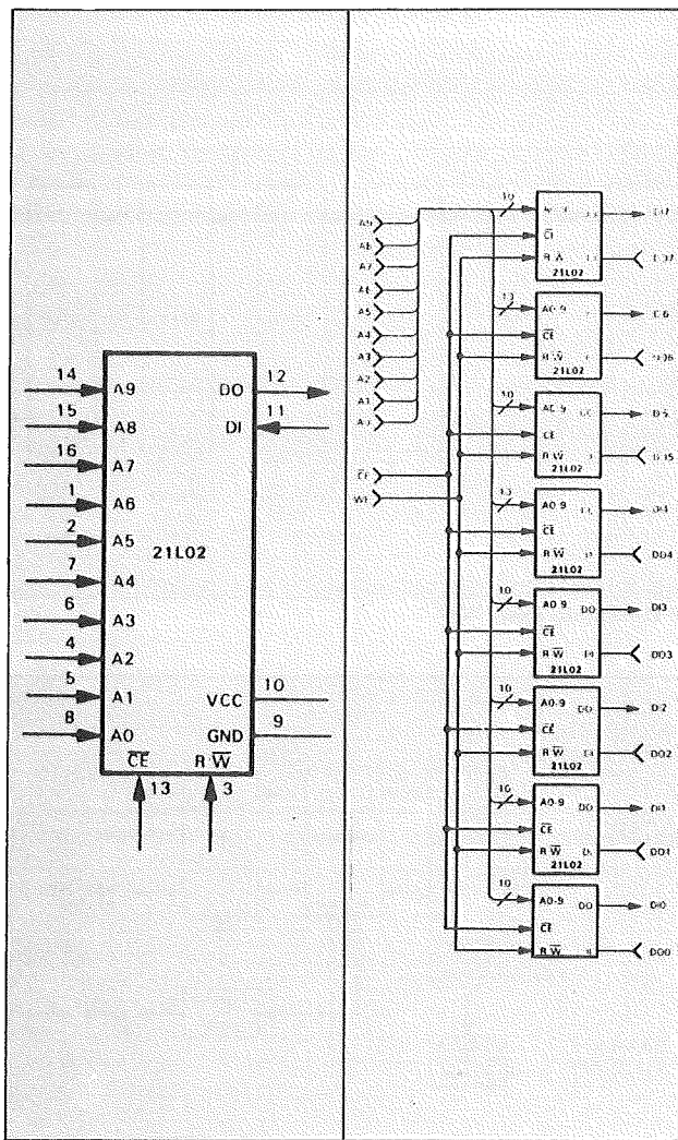
Figura 1A — Configuração dos Pinos Figura 1B — Organização 1K x 8 Utilizando Oito 21L02
