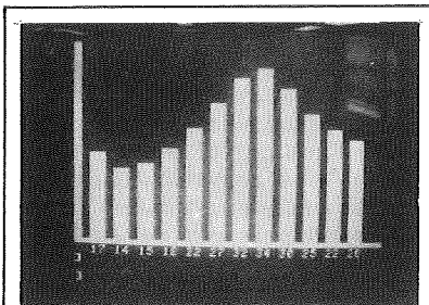
FIGURA 3 — Gráfico de barras ou histograma para o exemplo 2. temperatura X hora
