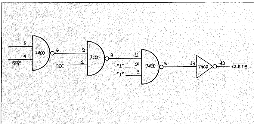
FIGURA 4B — Geração do sinal CLKTB (pulso de clock para deslocamento de memória)
