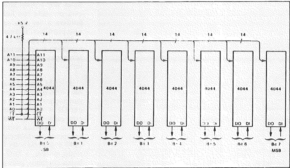
Figura 3B — Organização 4K x 8 Utilizando Oito 4044
