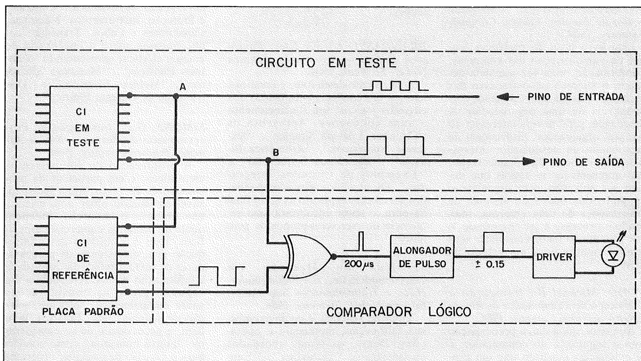
FIGURA 1 — Diagrama de um comparador lógico em teste
