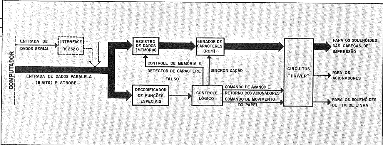
FIGURA 1 — Diagrama em bloco geral
