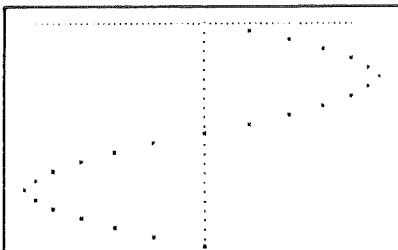
FIGURA 1 — Gráfico de uma senóide tirado em impressora.
