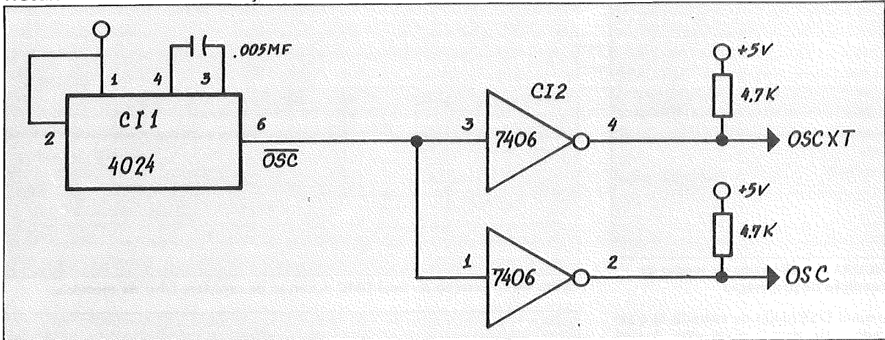
FIGURA 2A — Gerador de clock de 100 KHZ
