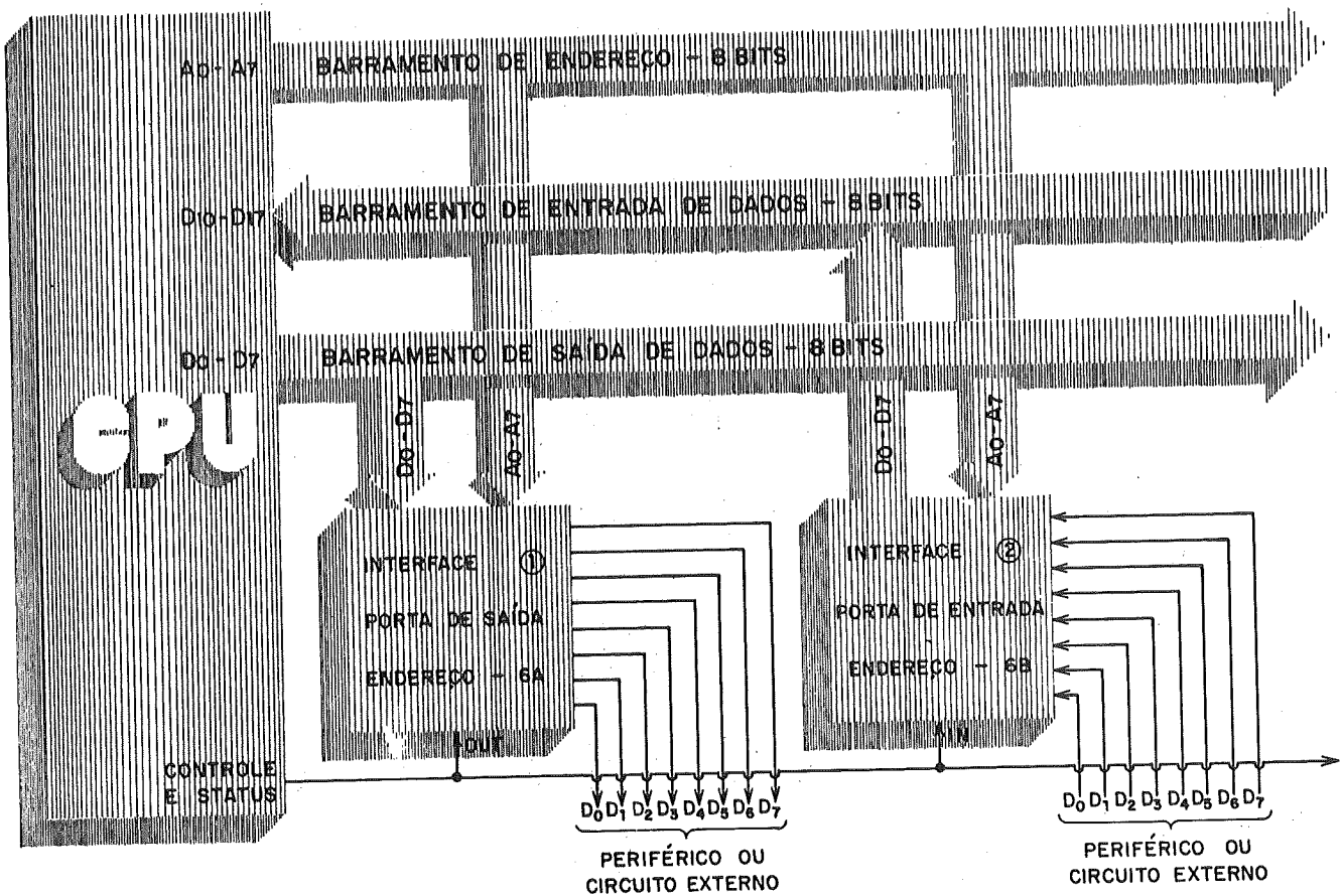
FIGURA 1 – DIAGRAMA EM BLOCO DE UMA CPU COM UMA PORTA DE SAÍDA 6A E UMA PORTA DE ENTRADA 6B
