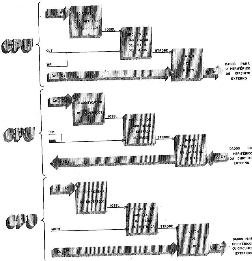
FIGURA 1 – DIAGRAMA EM BLOCO DE UMA CPU COM UMA PORTA DE SAÍDA 6A E UMA PORTA DE ENTRADA 6B
