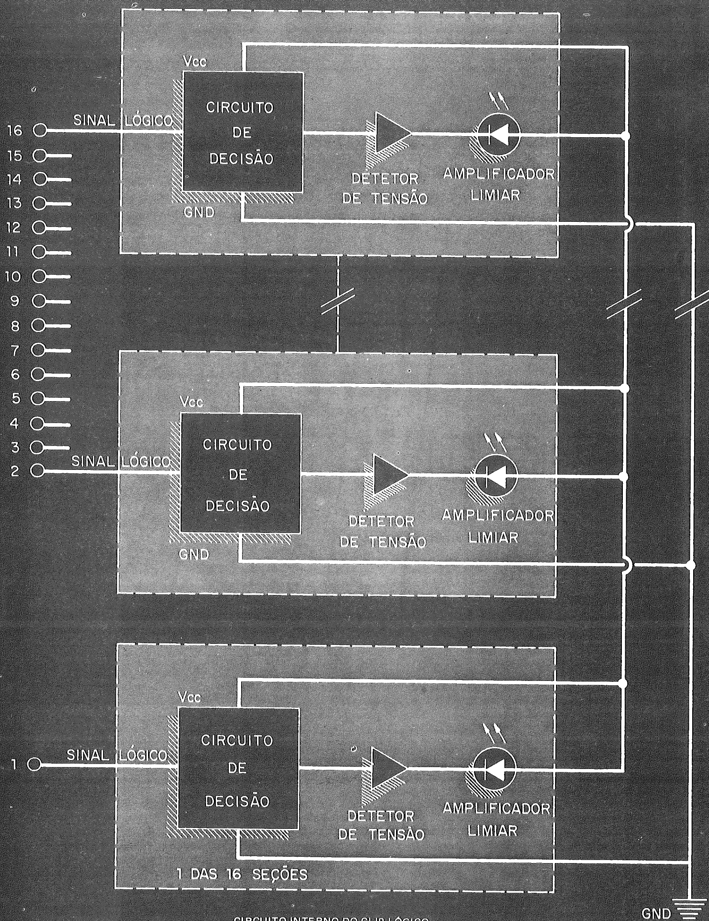
CIRCUITO INTERNO DO CLIP LÓGICO FIGURA 2
