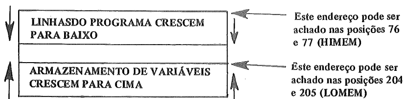
FIGURA 3 – MAPA DE MEMÓRIA DE PROGRAMA EM INTEGER BASIC
