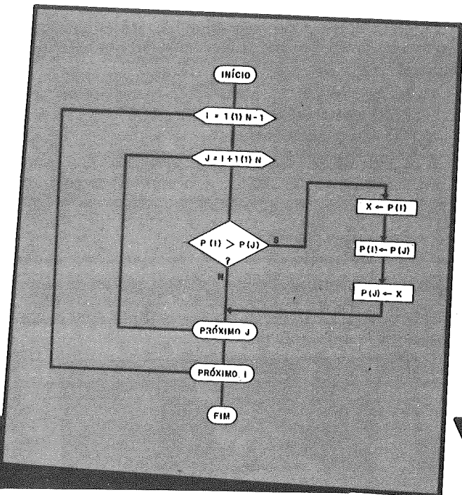
FIGURA 1 – ALGORITMO DE ORDENAÇÃO CRESCENTE DO VETOR P DE n ELEMENTOS
