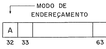
FIGURA 1 - FORMATO DA METADE DIREITA DO PSW DO 370-XA
