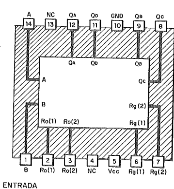
CONFIGURAÇÃO DOS PINOS DO CI 7490
