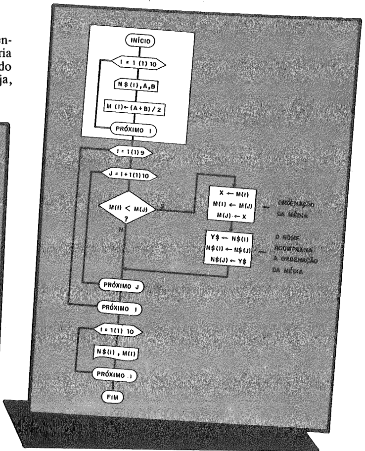
FIGURA 2 – ALGORITMO PARA LISTA DE ALUNOS NA ORDEM DECRESCENTE DAS MÉDIAS, POR ISTO O TESTE DE ORDENAÇÃO É M(I) < M(J)
