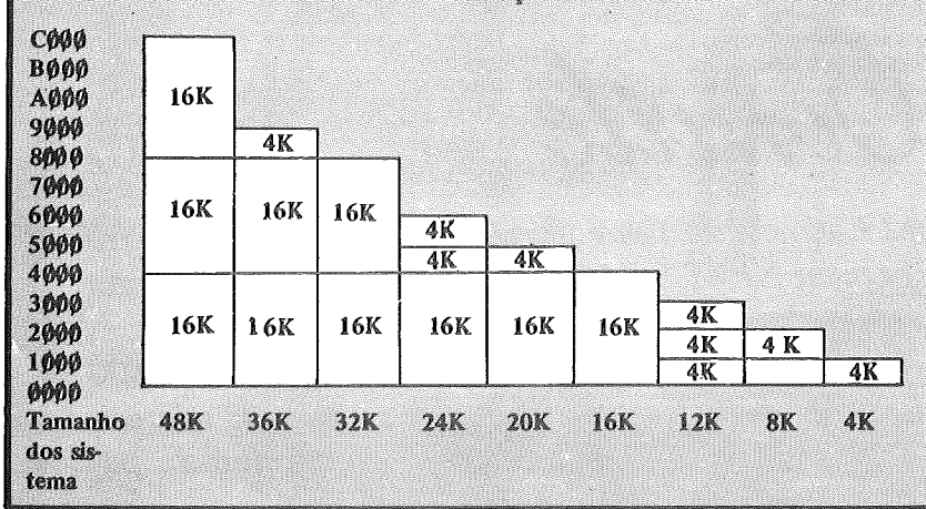
FIGURA 5 – CONFIGURAÇÃO DE MEMÓRIA
