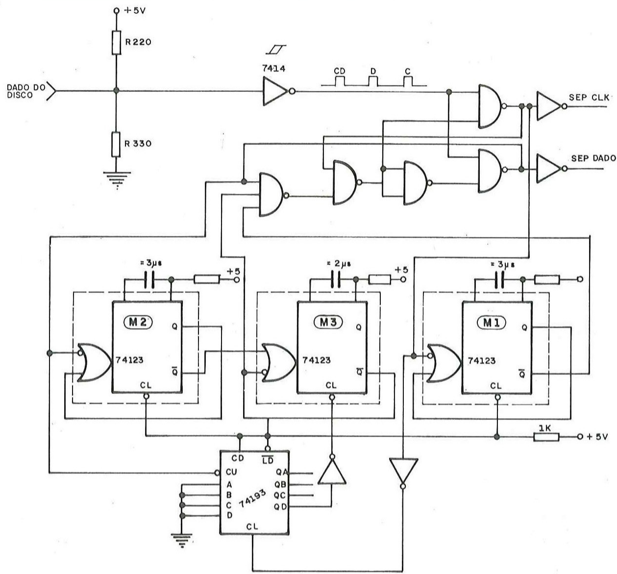
FIGURA 7 — SEPARADOR DE DADOS PARA O C. I. WD 1771, UTILIZANDO MONOESTÁVEIS
