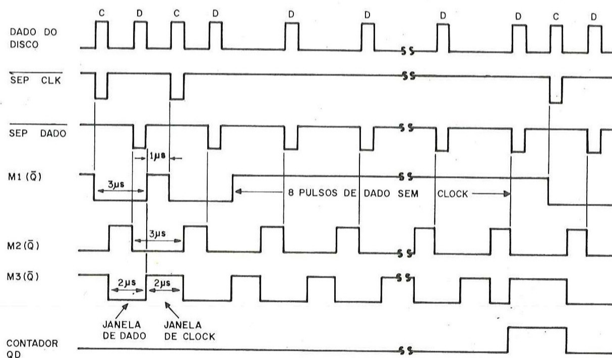
FIGURA 8 — DIAGRAMA DE TEMPOS DO SEPARADOR COM MONOESTÁVEIS
