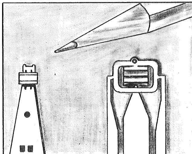
FIGURA 1 – COMPARAÇÃO DE TAMANHO ENTRE UMA CABEÇA WINCHESTER TRADICIONAL (À DIREITA) E UMA CABEÇA DE FILME-FINO.
