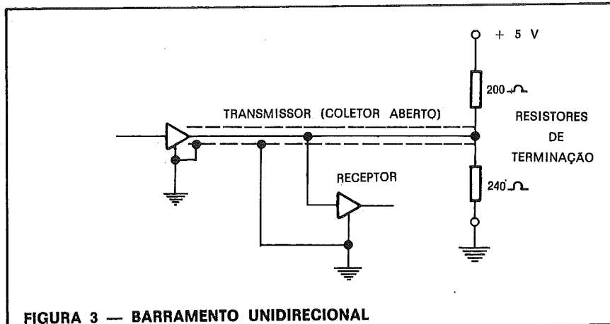
FIGURA 3 — BARRAMENTO UNIDIRECIONAL
