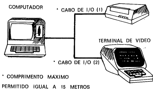
FIGURA 1 — PERIFÉRICOS LIGADOS DIRETAMENTE AO CONECTOR DE I/O, COMUNICAÇÃO EM PARALELO
