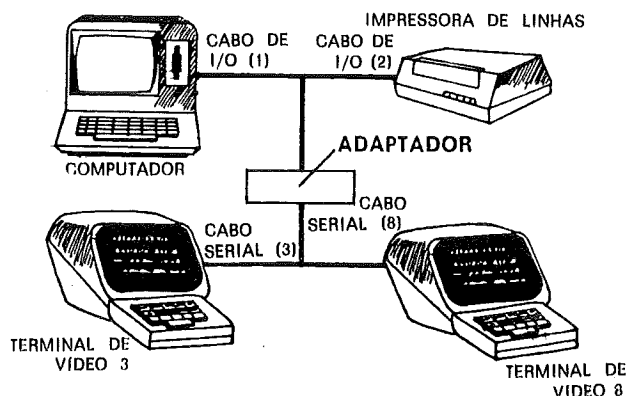
FIGURA 2 — SISTEMA COM TERMINAIS DISTRIBUÍDOS E IMPRESSORA LOCAL USANDO ADAPTADOR DE COMUNICAÇÃO
