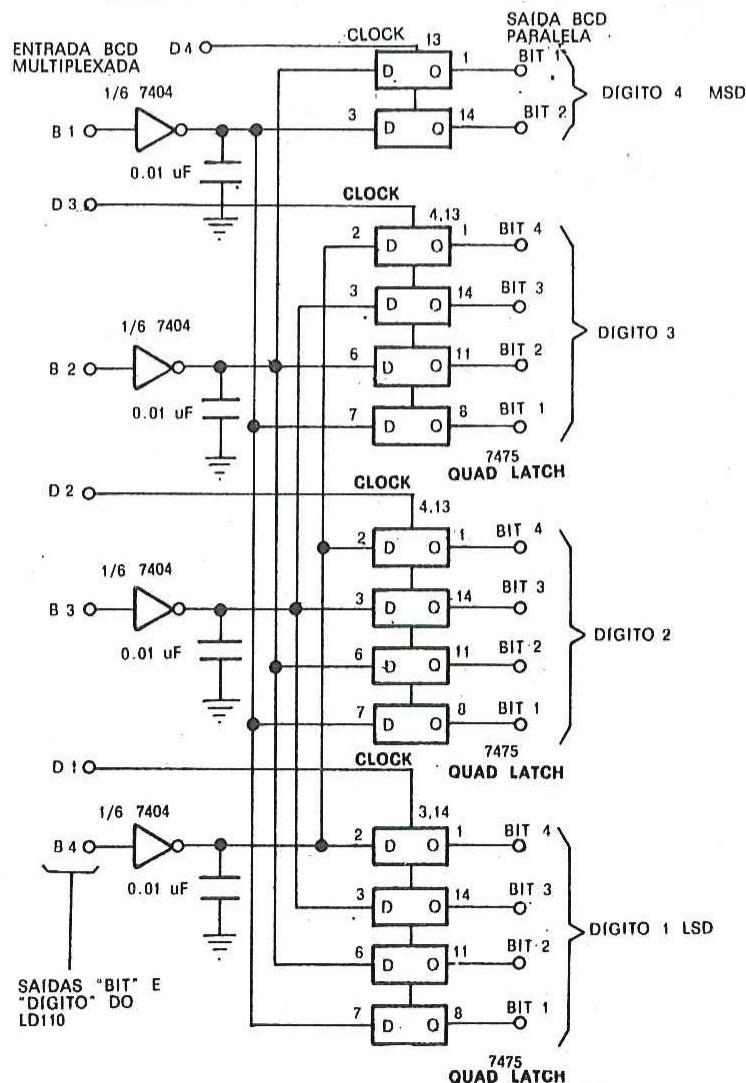
FIGURA 5 — REGISTROS PARA A SAÍDA PARALELA
