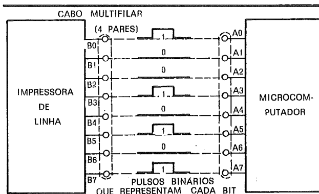
FIGURA 1 — LIGAÇÃO ESQUEMÁTICA DE UMA IMPRESSORA DE LINHA COM O MICROCOMPUTADOR
