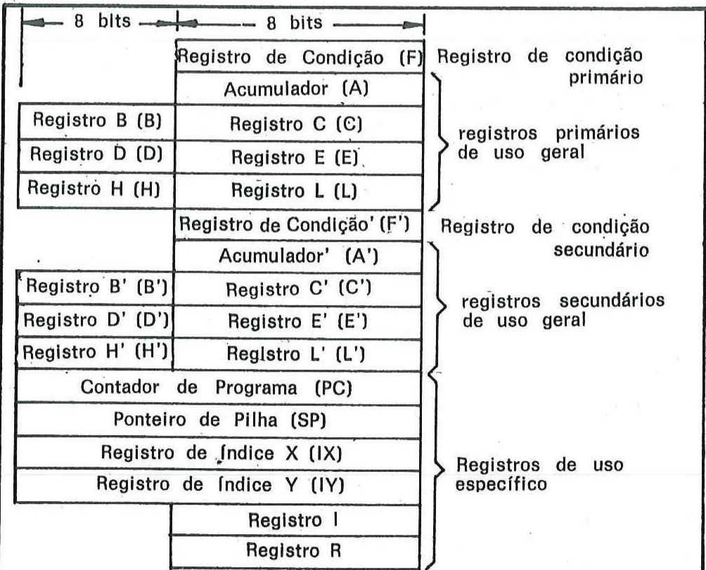
FIGURA 7 — MAPA DE REGISTROS DO Z-80
