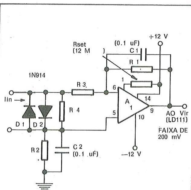
FIGURA 3 — AMPERÍMETRO DIGITAL
