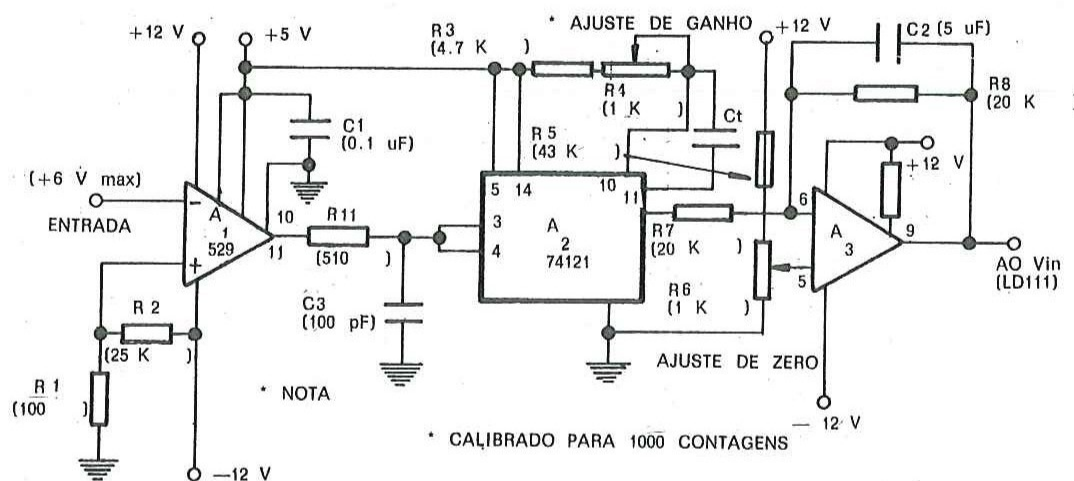
FIGURA 4 — FREQUENCÍMETRO DIGITAL
