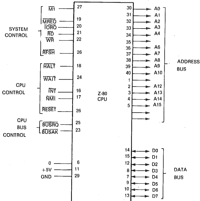
FIG. 7 — CONFIGURAÇÃO DE PINOS DO UPZ-80
