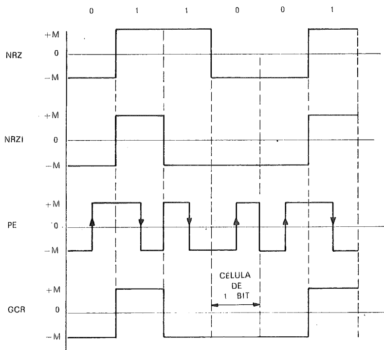
FIG. 4 — MÉTODOS DE CODIFICAÇÃO DA INFORMAÇÃO UTILIZADOS EM FITAS MAGNÉTICAS
