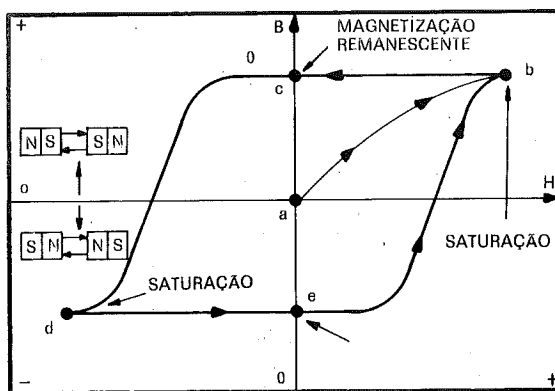
FIG. 1 — CURVA DE HISTERESE (e b c d e)
