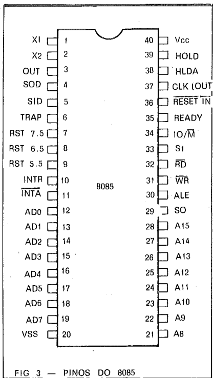
FIG. 3 — PINOS DO 8085
