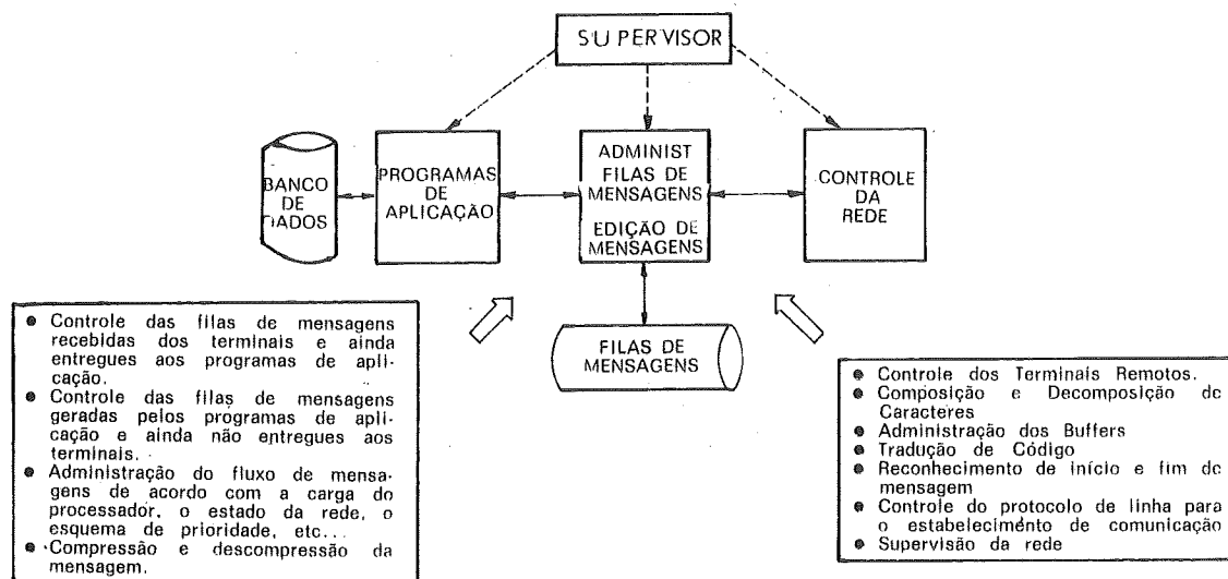
FIGURA 4 — FUNÇÕES DE UM SISTEMA DE TELEPROCESSAMENTO REALIZADAS POR "SOFTWARE"
