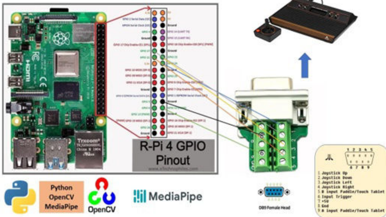
Fig. 1 - Lo schema di collegamento
