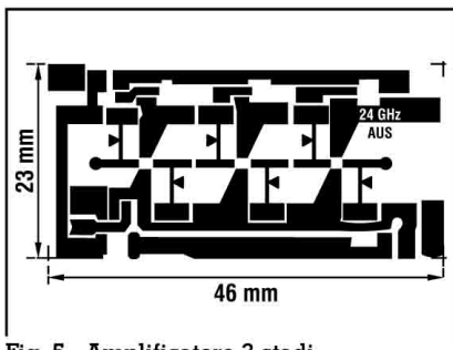
Fig. 5 - Amplificatore 3 stadi
