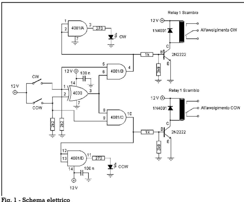
Fig. 1 - Schema elettrico
