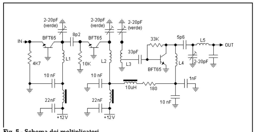
Fig. 5 - Schema dei moltiplicatori
