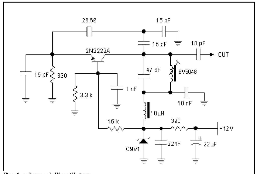
Fig. 4: schema dell'oscillatore
