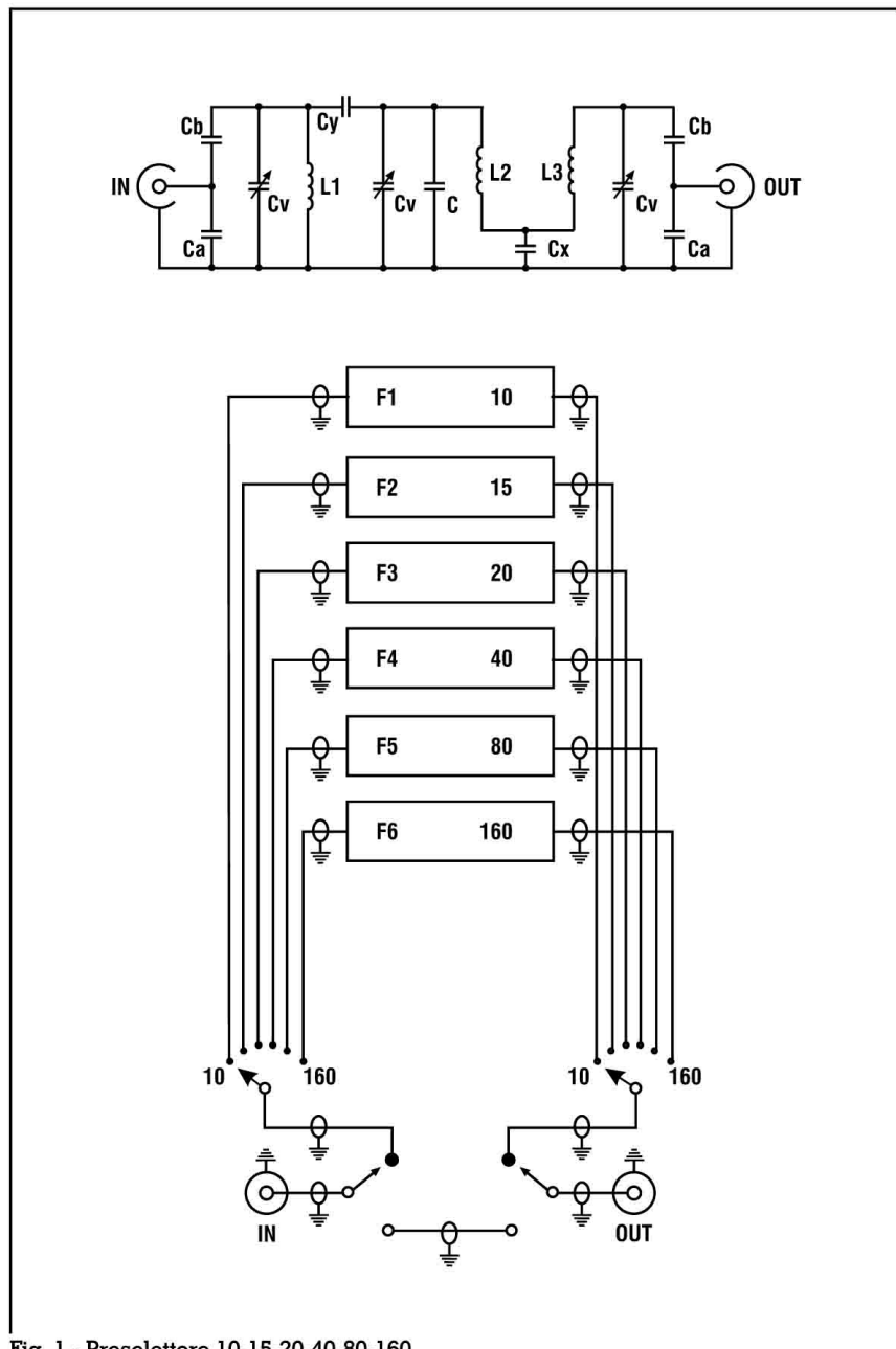
Fig. 1 - Preselettore 10-15-20-40-80-160
