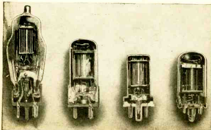
TYPE 6J7G
