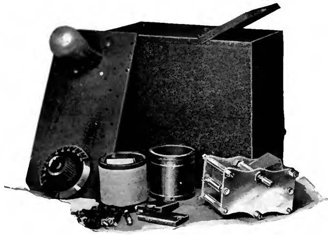
THE GENERAL INSTRUMENT R. F. UNIT
