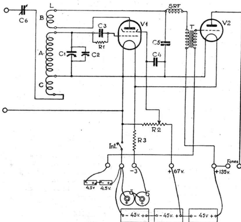
Fig. 1 — Circuito do Receptor para Baterias
