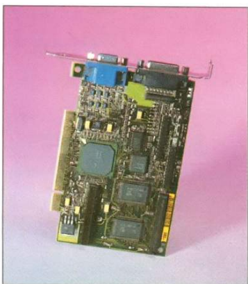
Matrox Mystique: Noch die Eierschalen hinter den Ohren.
