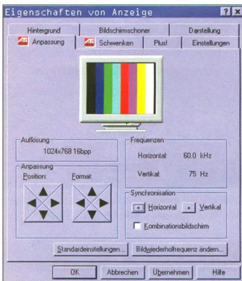
Die ATI-Karten klinken sich mit erweiterten Optionen ins Einstellungs-menü ein
