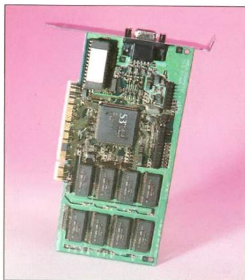
ELSA Victory 3D: eine der ersten fertigen 3D-Beschleunigerkarten auf dem Markt
