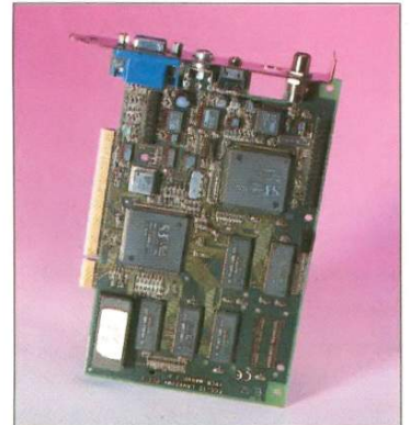
Miro Media 3D: S3-Virge als Herz der Karte, Zusatzanwendungen möglich.
