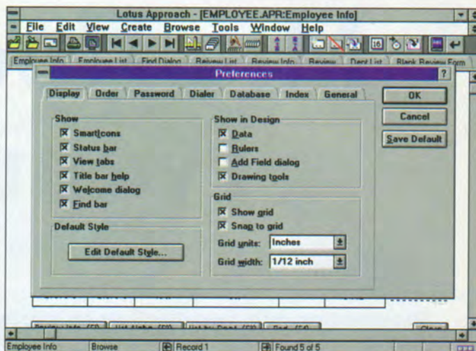
Το παράθυρο των ρυθμίσεων μας επιτρέπει να προσδιορίσουμε τόσο τη γενική εμφάνιση του Approach όσο και την εμφάνιση του αρχείου που δουλεύουμε εκείνη τη στιγμή.
