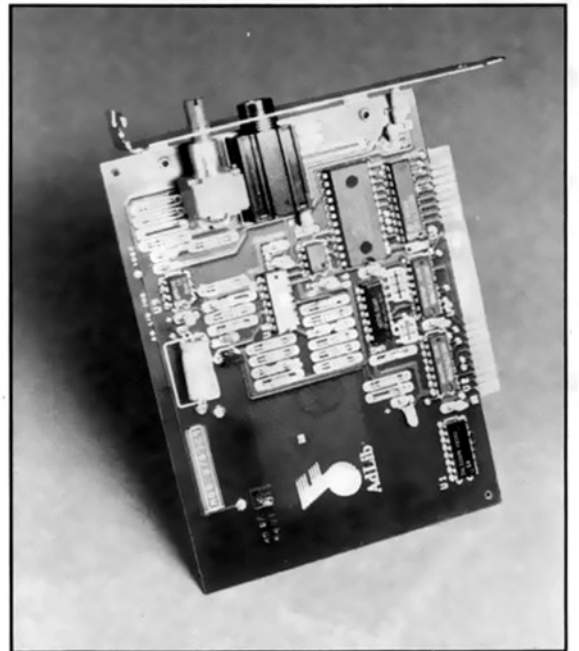
Η hardware προσωπικότητα του Ad Lib. Διακρίνεται το ρυθμιστικό της έντασης και η υποδοχή των ακουστικών.
