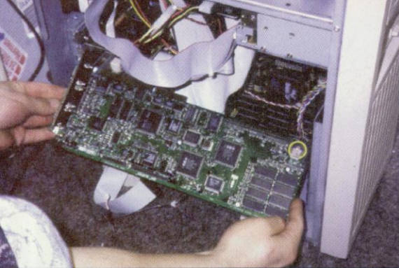
Der 3DO-Blaster ist mit edlen Bauteilen nur so bestückt
