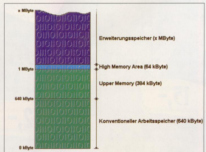
Die "Landkarte" des PC-Speichers mit den vier unterschiedlichen Speicherregionen
