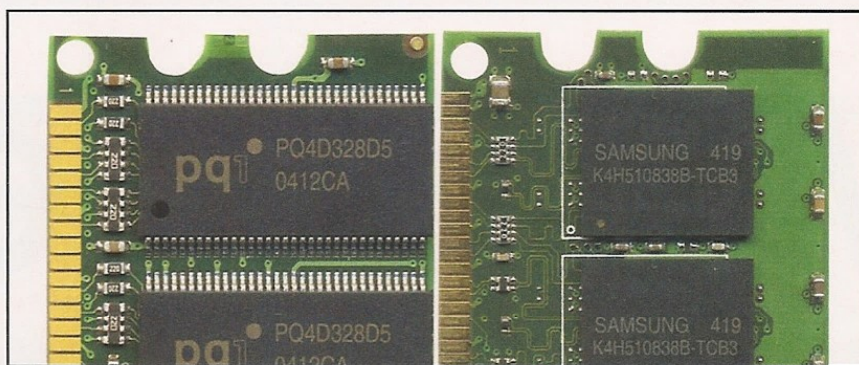
Memória DDR (à esq.) é retangular e a DDR2 (à dir.) é quadrada. Diferença ocorre em função do terminal de contato
