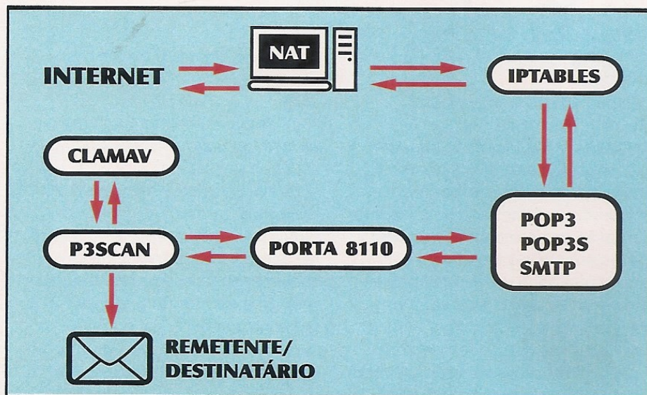
Sistema de Proxy Mail utiliza os recursos Iptables e software de antivírus pelo caminho descrito no gráfico acima
