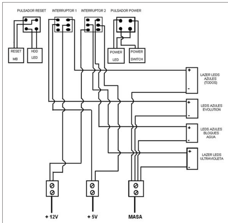
Este esquema gráfico nos va a permitir hacernos una idea muy aproximada de la instalación y cableado necesario para dar servicio a las luces incorporadas en nuestro mod.
