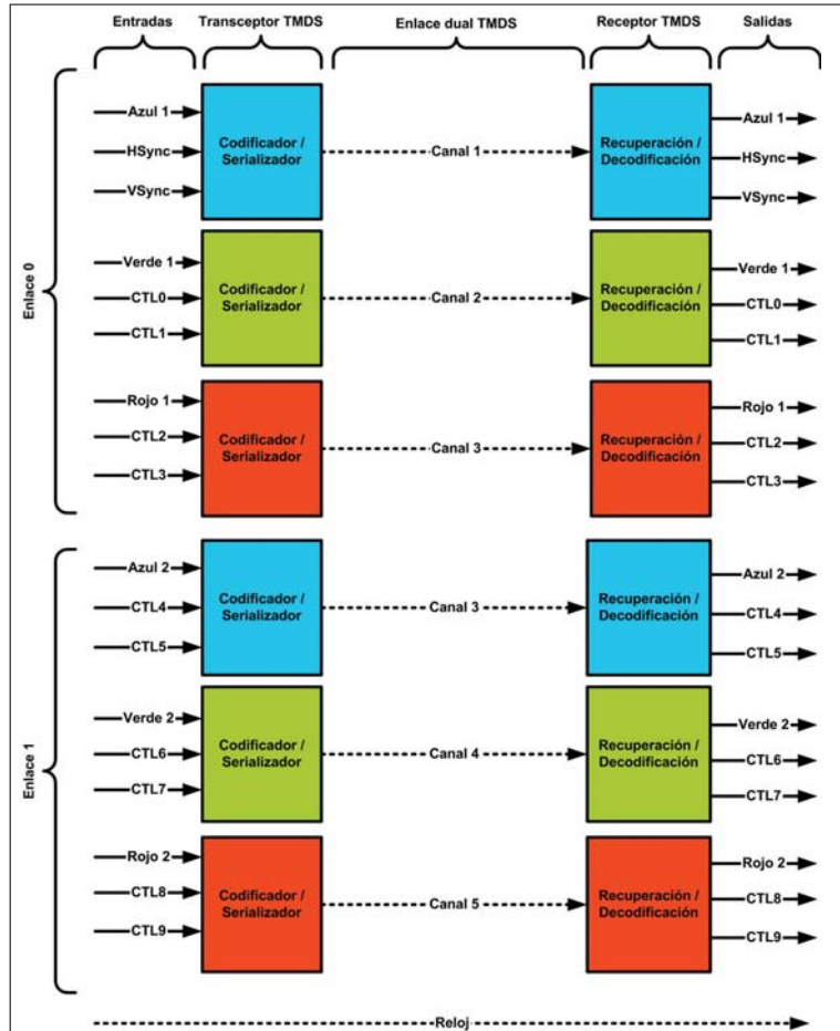
Esquema algo simplificado de cómo se organiza el envío de las señales entre dos dispositivos. En éste, se representan los canales rojo, verde, azul y las señales de control. Como comentamos a lo largo de este reportaje, la señal de reloj es única para ambos enlaces y cada uno de ellos dispone de tres canales independientes.
