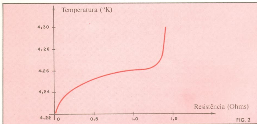
Gráfico da Temperatura × Resistência para o mercúrio. Observe que a partir de 4,26 °K a resistência do mercúrio decresce acentuadamente, chegando a zero em 4,22 °K.
