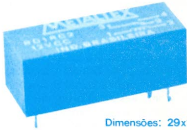
Dimensões: 29x11,5x11mm
