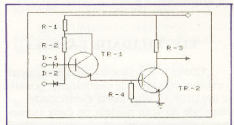
Fig. 3 - Circuito eletrônico de uma porta NAND. TR-1 e TR-2 são tipo 2N2222. Os diodos são do tipo 1N914 e os resistores de 2.000 ohms, 1/8 de watt. Bastam entre uma e três centenas destas portas a Máquina Speculatrix MSX 3.0.
