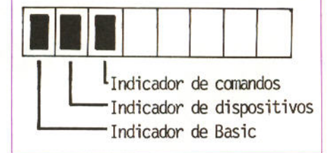
Figura 5 - Bytes de atributos dos slots (SLTATR)
