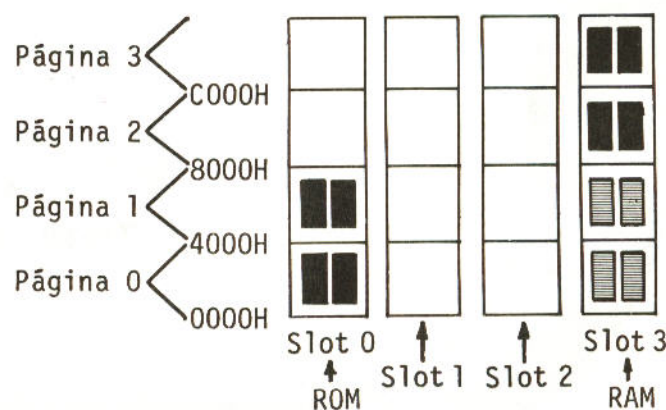
Figura 2 - Configuração de memória do HOTBIT 1.1 ou 1.2
