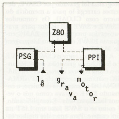
Figura 6 — Esquema do hardware de acesso ao cassette.
