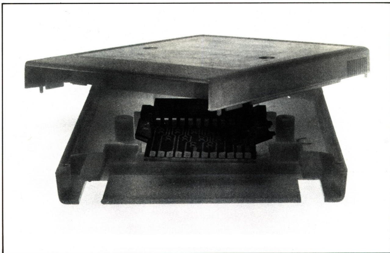
O cartucho de videogame por dentro, mostrando o circuito integrado, os pinos de encaixe e o pente conector (Cartucho Vidgame, fabricado pela Activision).
