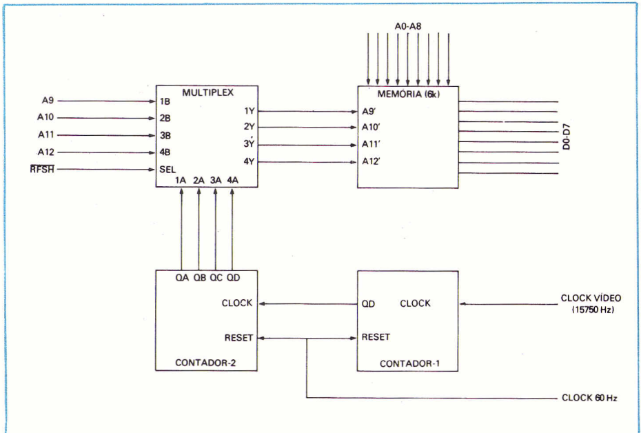
Figura 3 — Diagrama de blocos do circuito de alta-resolução.
