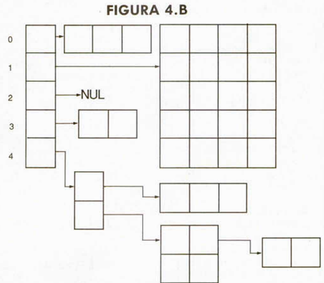
Fig. 4: Creación de estructuras. A/ Matrices multidimensionales. B/ Matrices de punteros.
