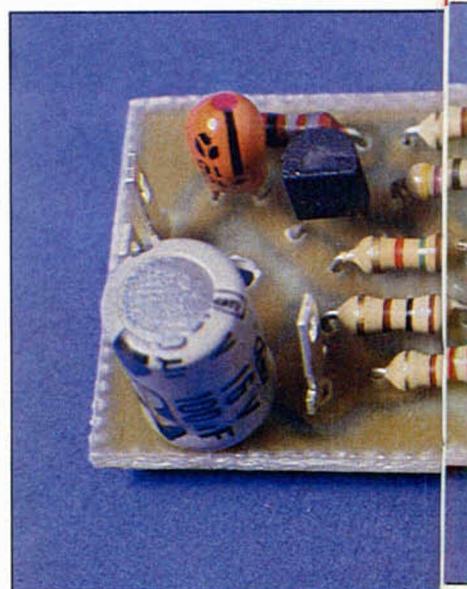
Aspecto final de la tarjeta una vez montada la totalidad de los componentes.
