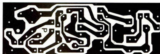
Fig. 2. Cara de pistas de la tarjeta a tamaño real.
