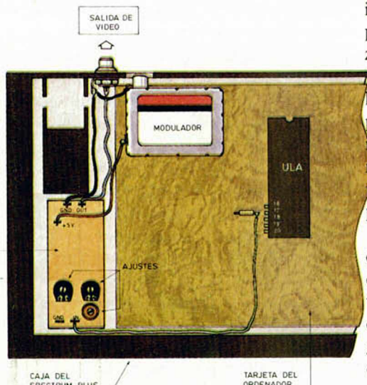
Fig. La tarjeta del amplificador de vídeo se aloja en el interior de la caja del Spectrum Plus tal como se muestra, soldando en los puntos indicados.
