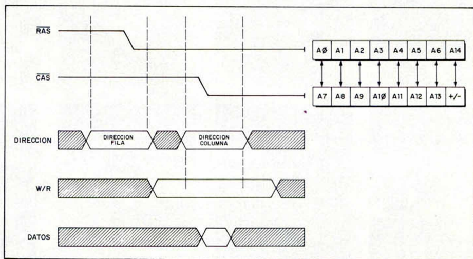
Diagrama de tiempos de la RAM dinámica TMS-4532. (Fig. 3).
