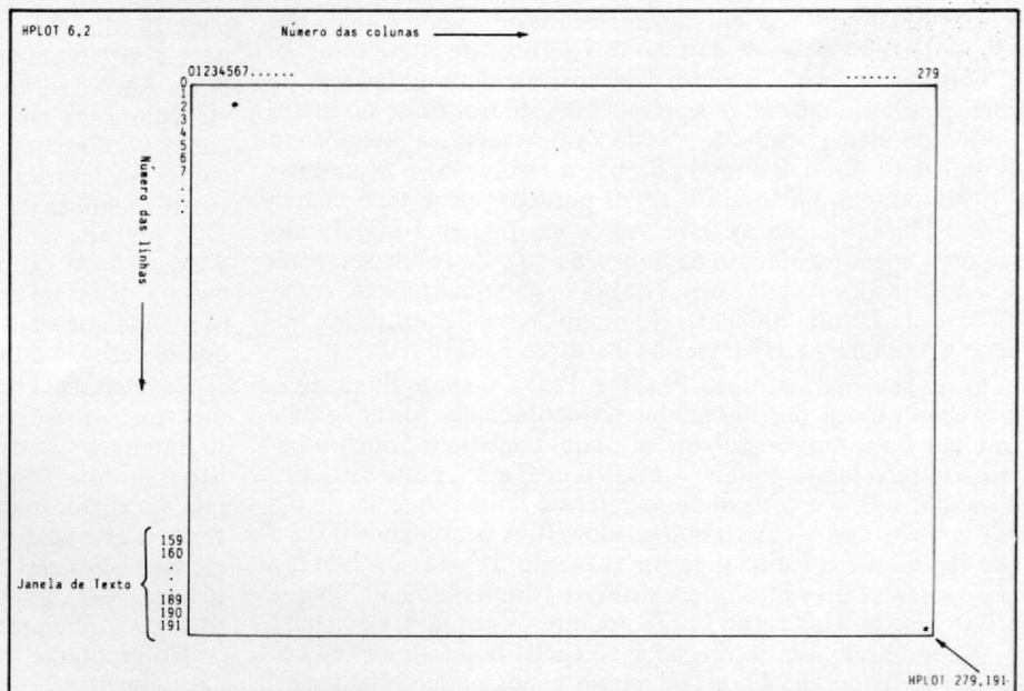
Figura 4 — Tela de alta resolução dos micros da linha Apple (as coordenadas aqui representam porções pequenas da tela que não dá para quadricular).
