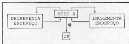
Figura 2: A flexibilidade do modo A
