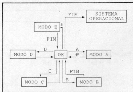
Figura 1: Organização do sistema
