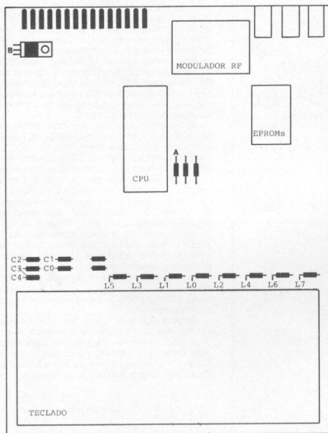
Figura 3 – Lay-out do TK85
