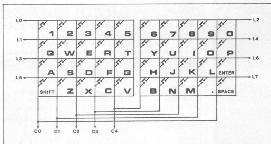
Figura 1 - Matriz do teclado
