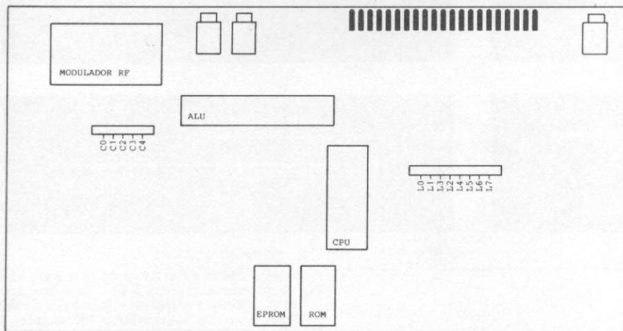
Figura 3 – Lay-out do TK85
