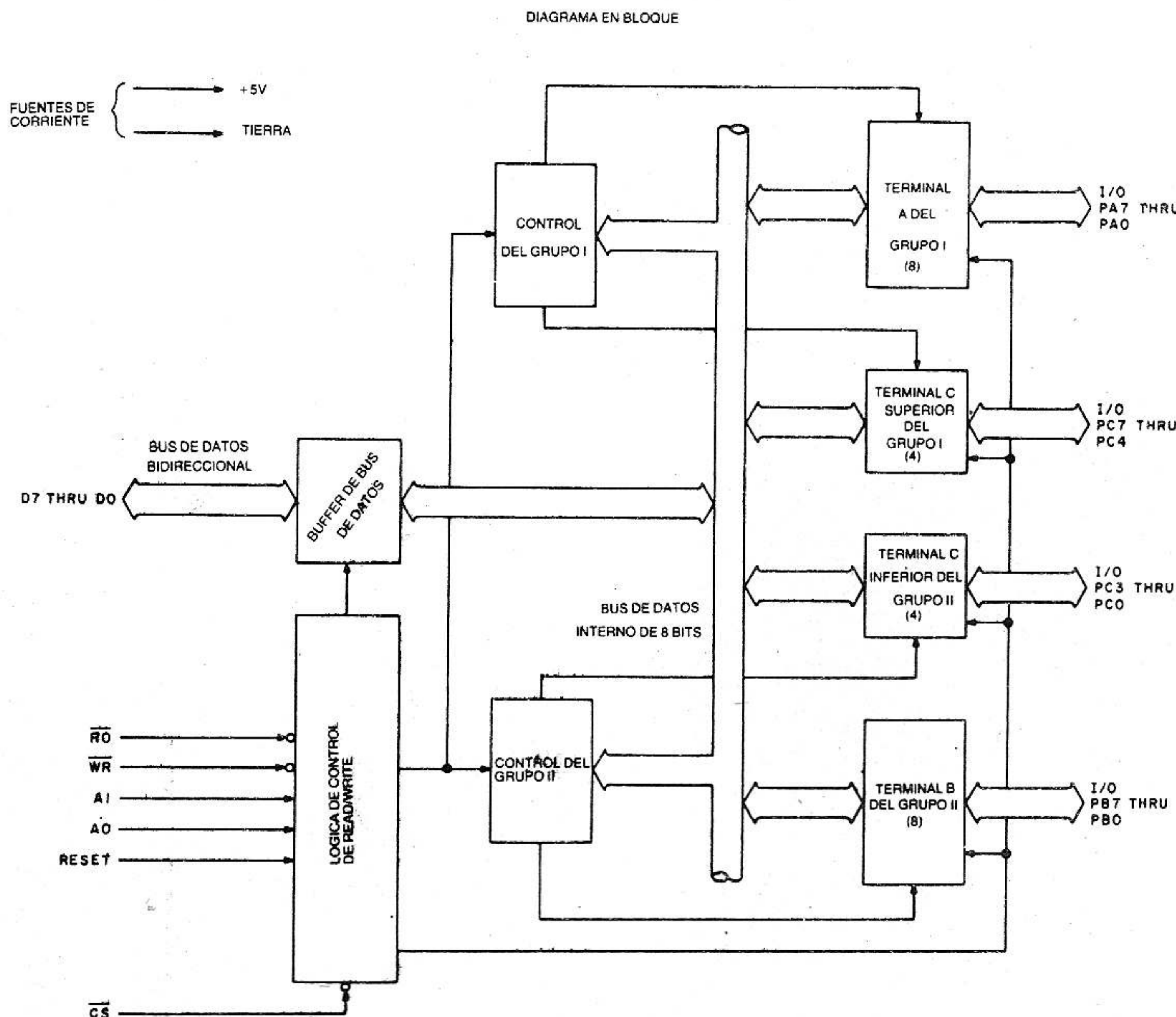
Fig. 1: Configuración y mobres de los pins de la interfase periférica programable del Intel 8255 y diagrama en bloque de sus partes funcionales.
