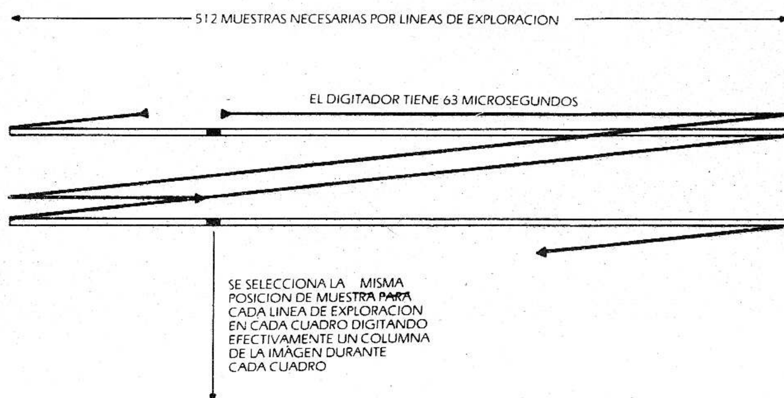
Fig. 8: Muestreando un único punto por línea de exploración, se puede completar la digitación de cada pixel en un plazo de 63 \mu\text{s} y los datos se producen a una velocidad bastante baja ( 15,7\text{K bytes/seg} ) para su transferencia a almacenamiento masivo.
