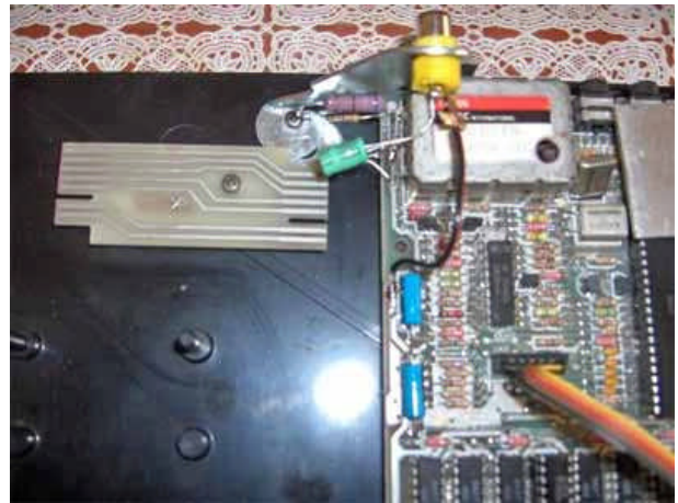
Imagen 5. Colocación del nuevo conector RCA
