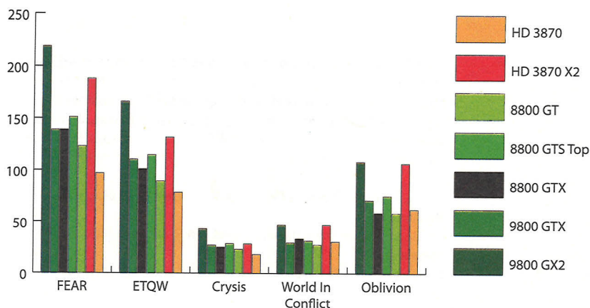
Jeux en 1920 par 1200, sans anti aliasing, afiltrage anisotrope 16x
