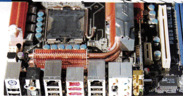
Les ports USB ont été espacés pour faciliter les branchements. Pas bête.
