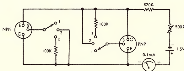
SWITCH POSITIONS : 1 : LEAKAGE 2 : SET FULL-SCALE 3 : \beta , 10-1000
